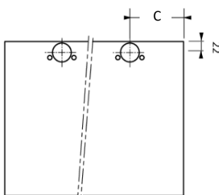
Porauskoodi S5
